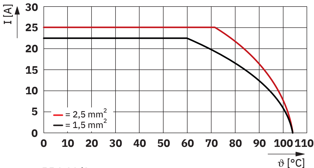
PRC 20/3... IEC 61535 / 2 conductors
