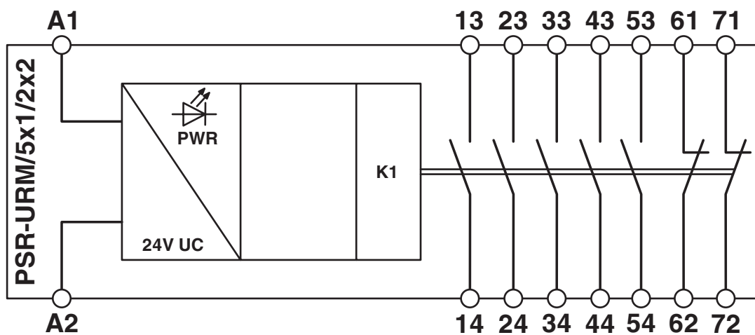
Kopplungsschema
