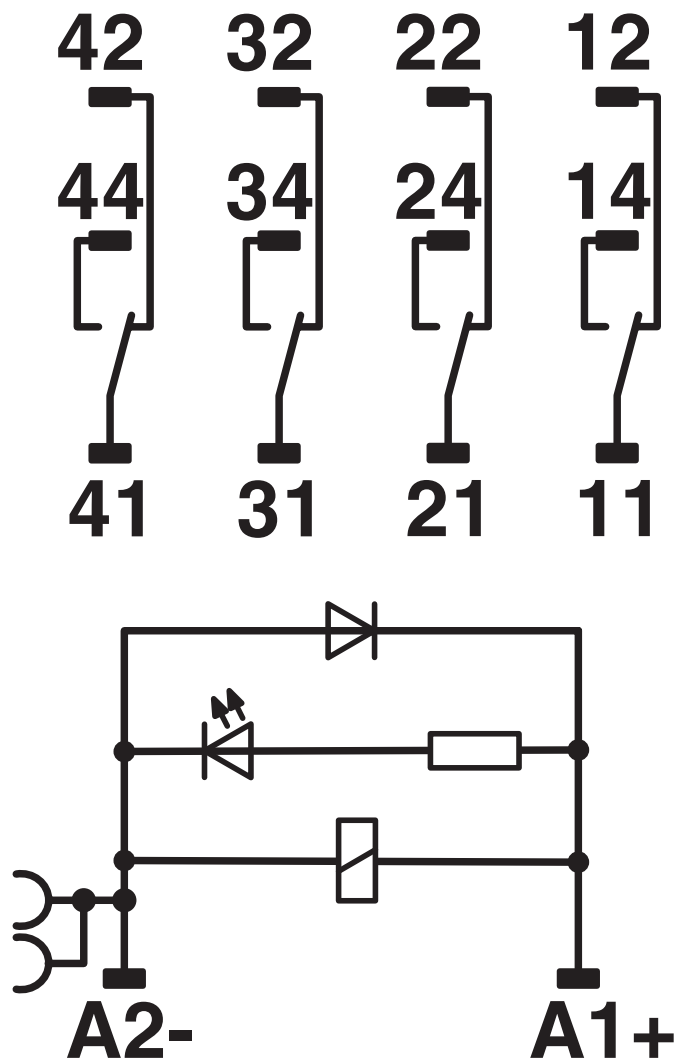
Kopplingsschema
