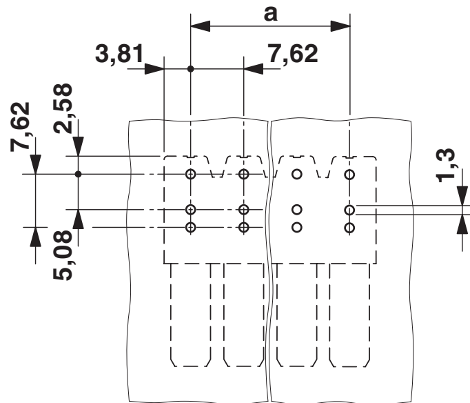
Borrplan/lödöns geometri
