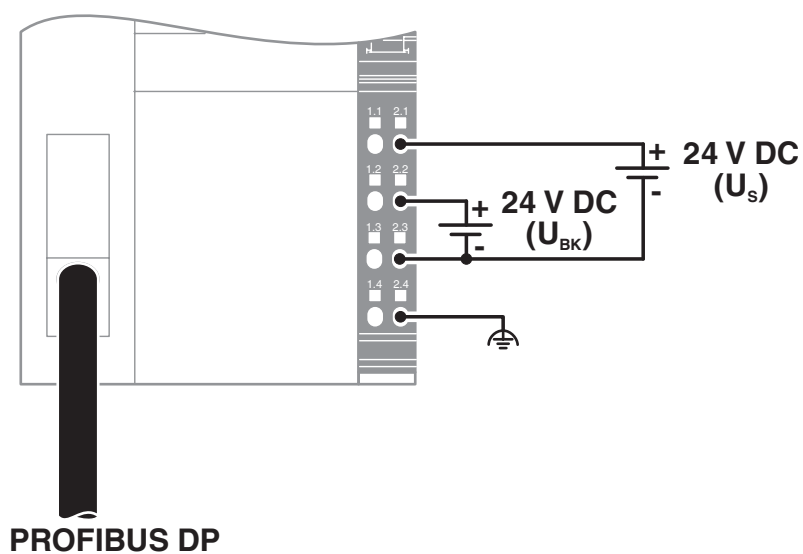
Disegno collegamento
