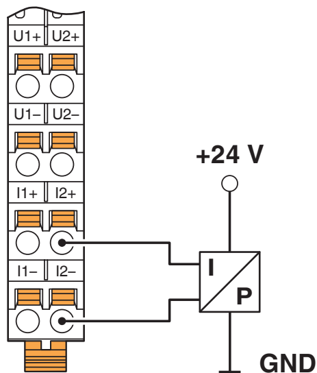
Sensore di pressione passivo su ingresso di corrente differenziale
