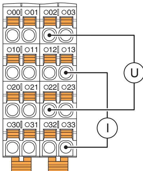
Disegno collegamento
