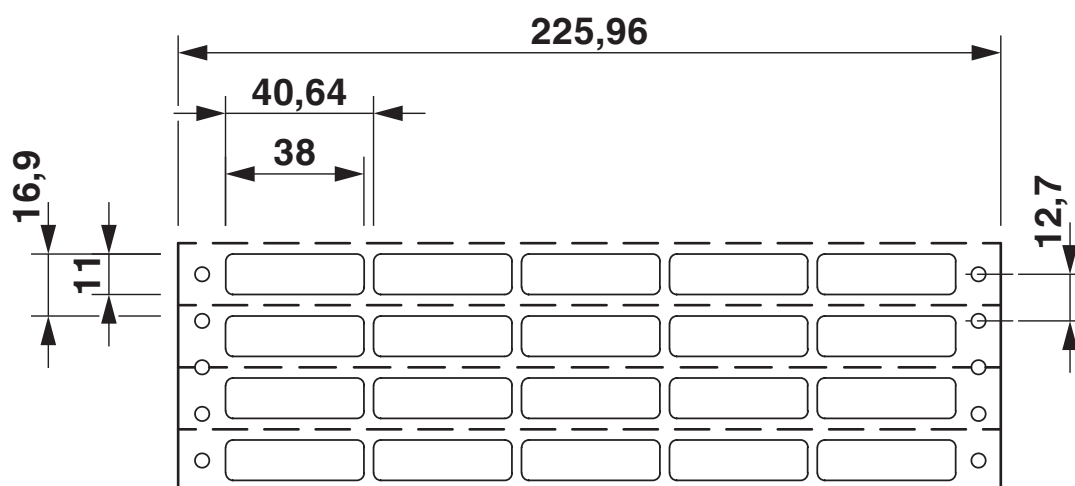
Disegno quotato
