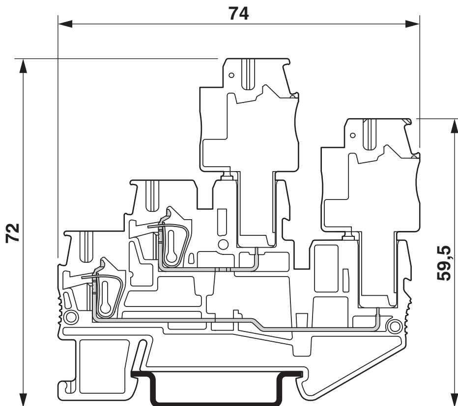
Disegno quotato
