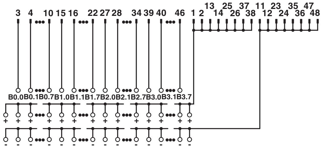
Schema di collegamento UM 45-FLK50/32IM/PLC
