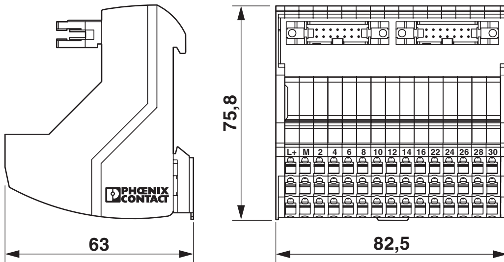
Disegno quotato
