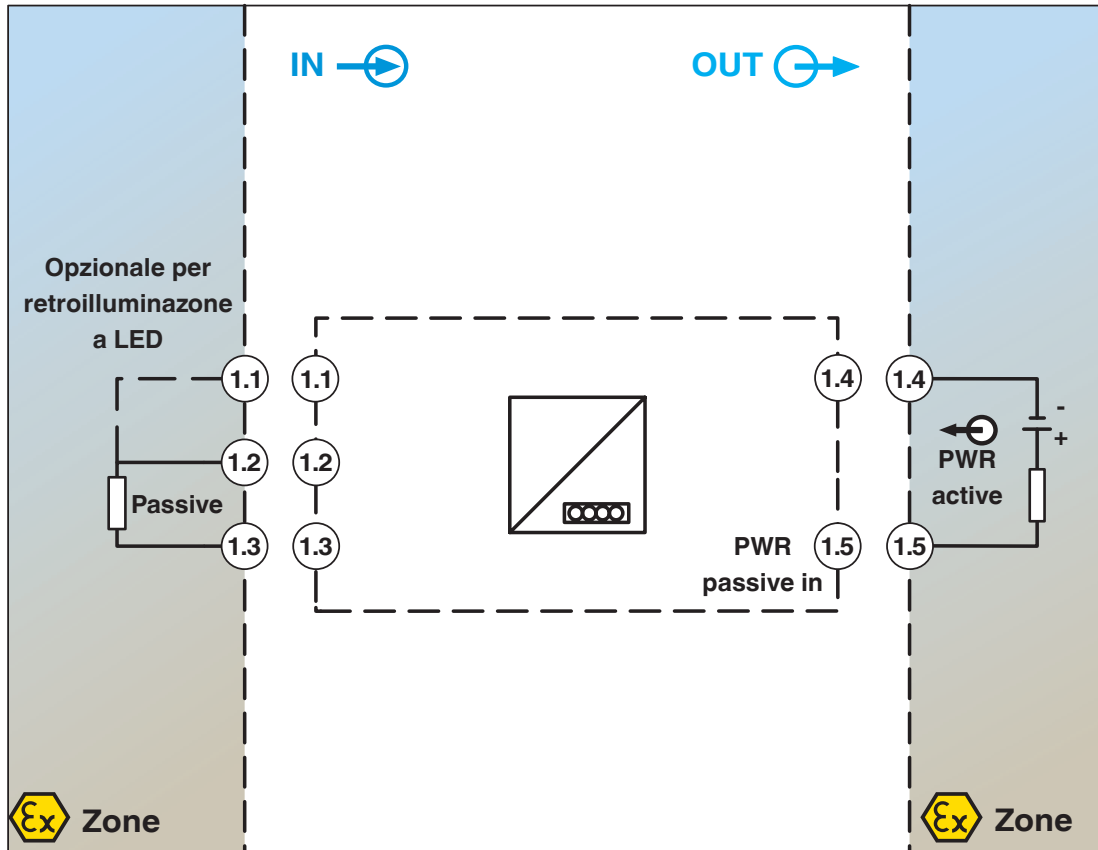
Diagramma a blocchi FA MCR-EX-DS-I-I-OLP
