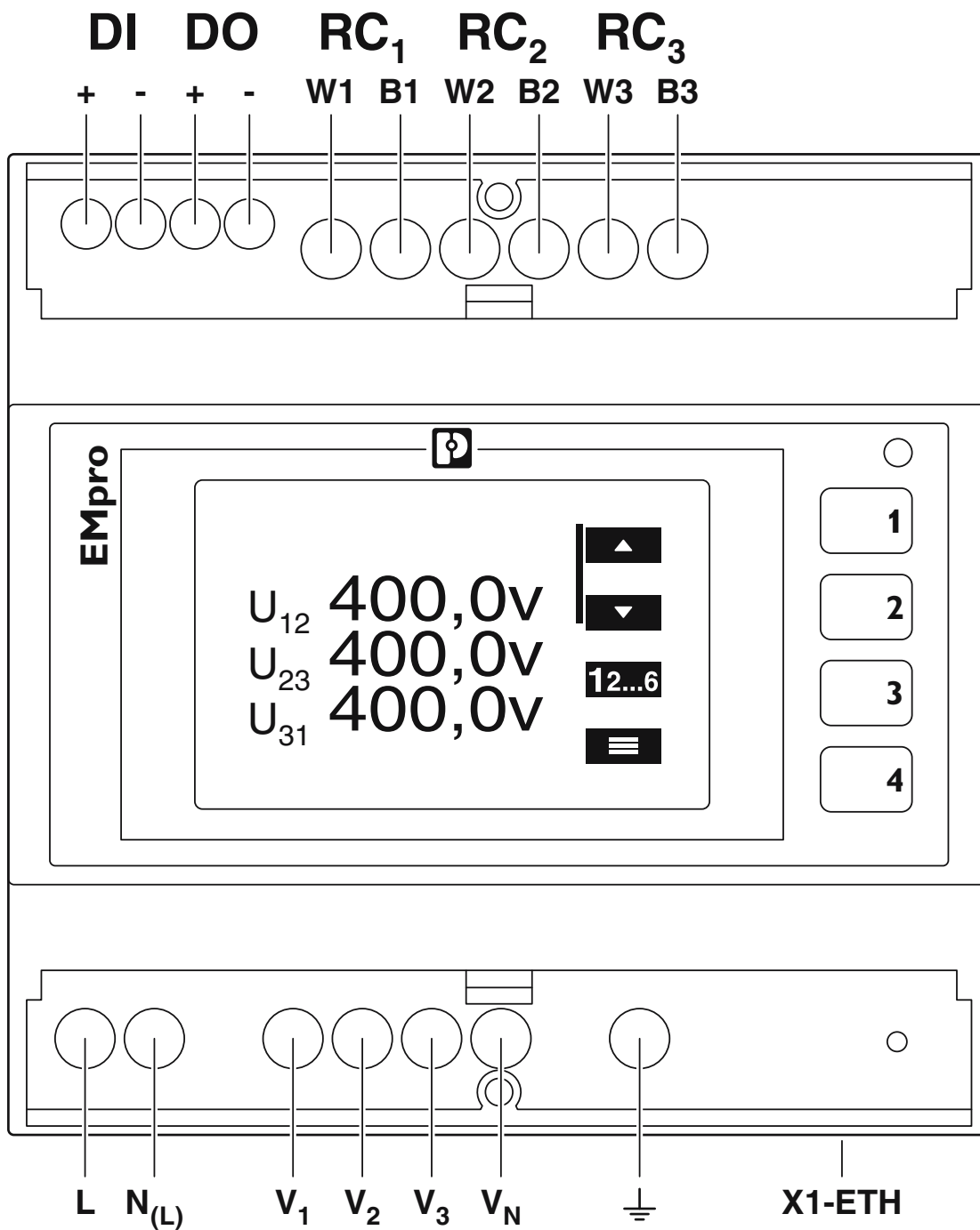
Disegno collegamento
