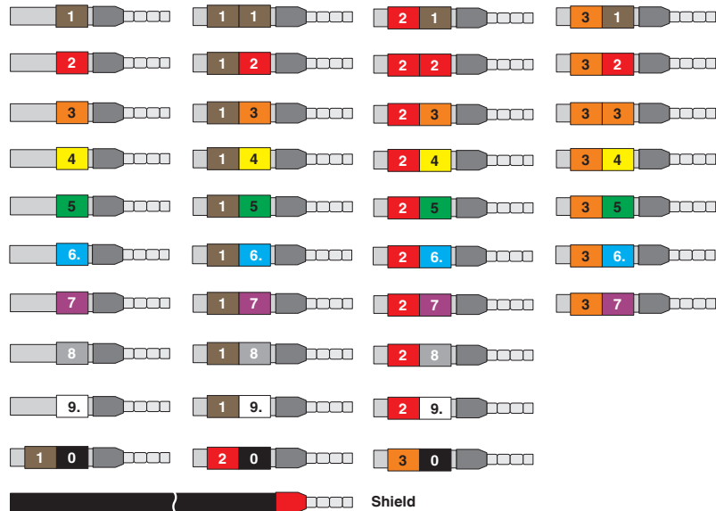
Disegno schema
