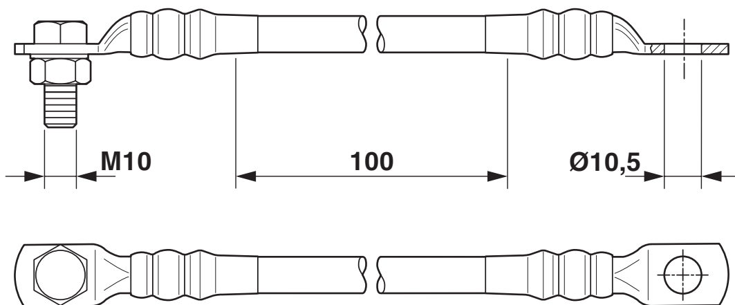
Disegno quotato
