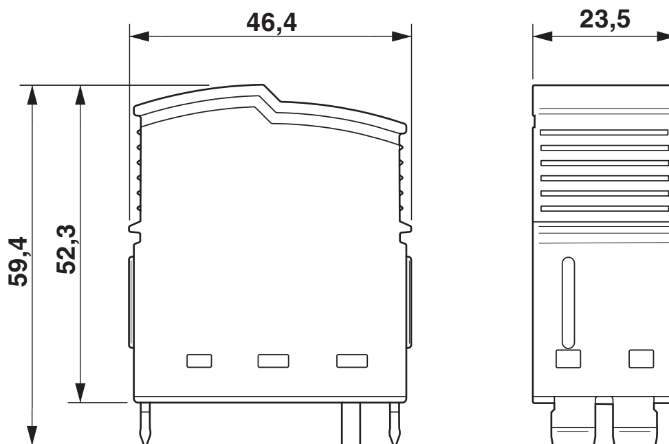
Disegno quotato
