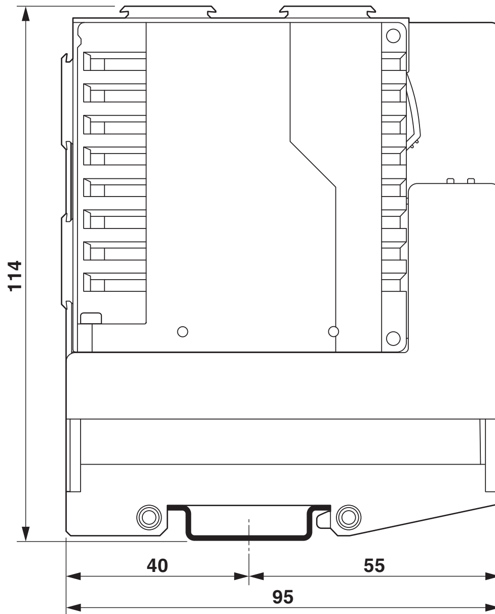
Disegno quotato
