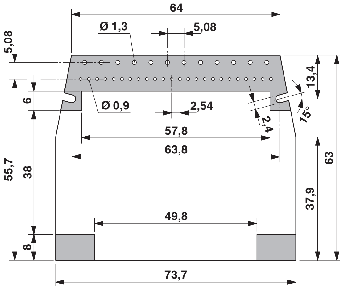
Disegno quotato
