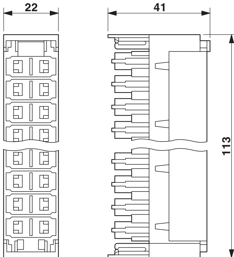
Disegno quotato
