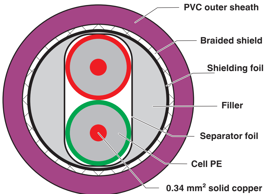
Disegno schema
