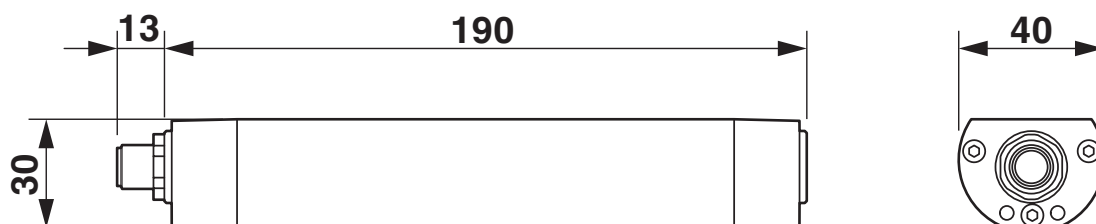
Disegno quotato
