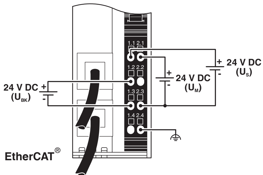
Disegno collegamento
