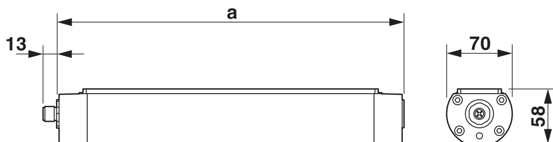
Disegno quotato
