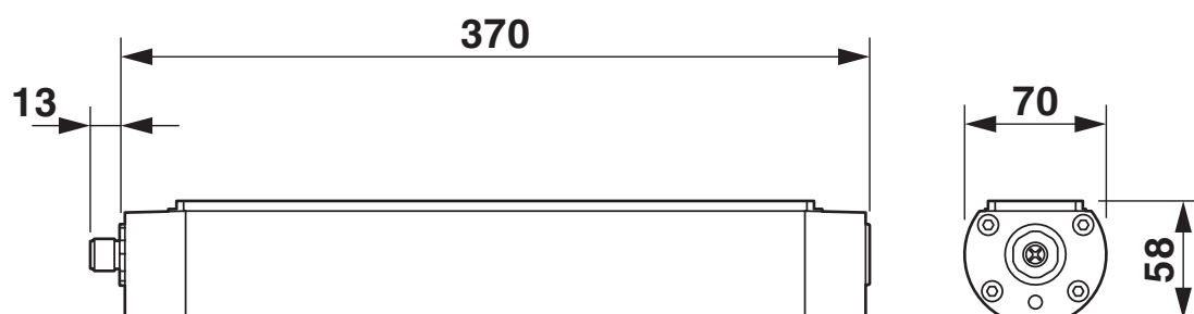
Disegno quotato
