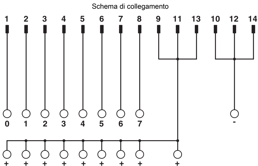
Schema di collegamento VIP-2/.../FLK14/8P/PLC
