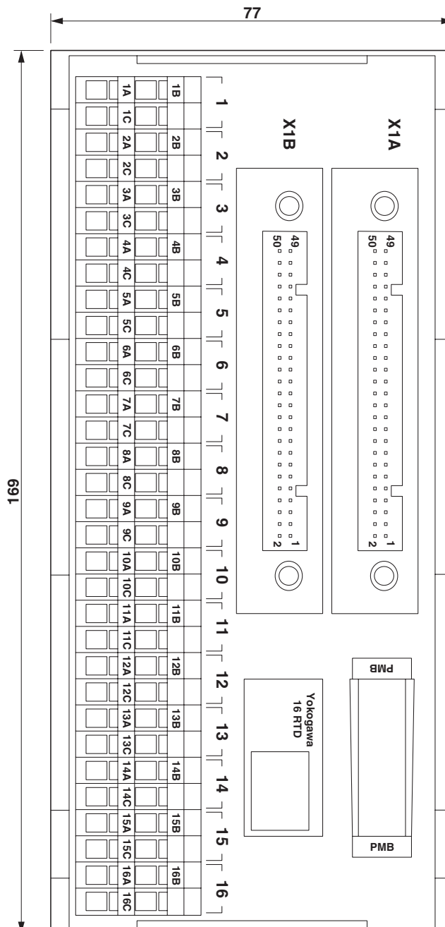
Disegno quotato
