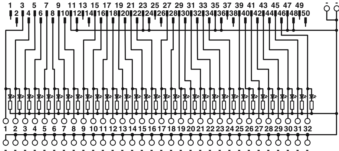
Disegno collegamento
