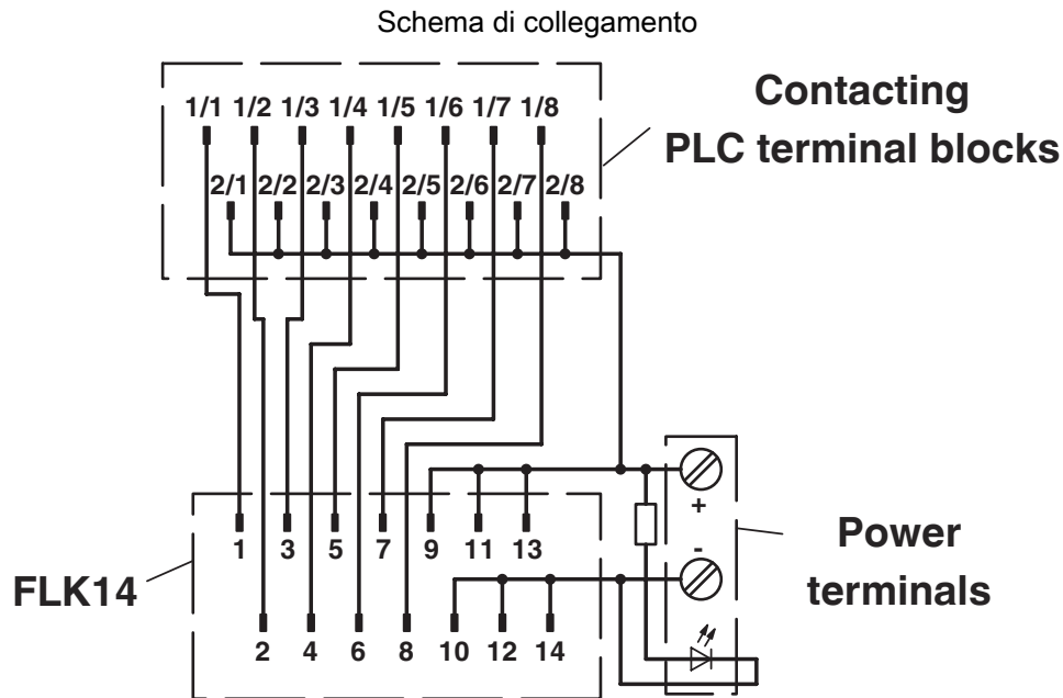
Schema di collegamento PLC-V8/FLK14/IN
