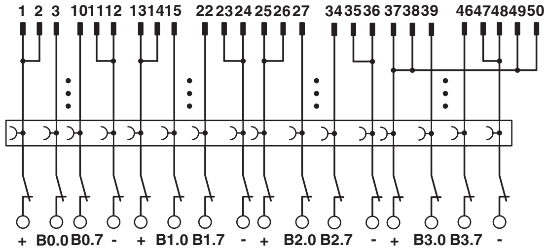
Schema di collegamento FLKM 50/KDS3-MT/PPA/PLC
