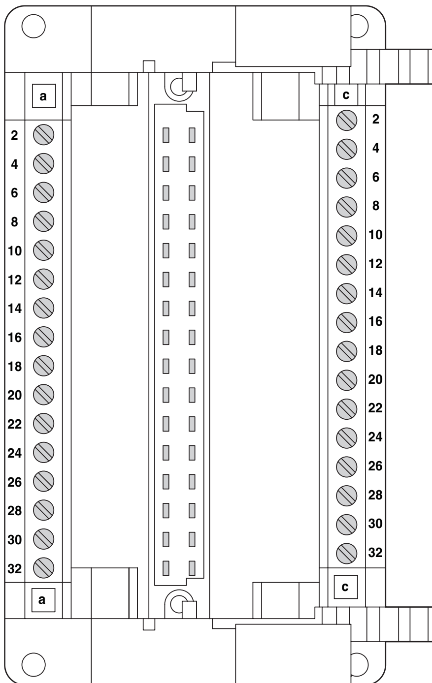
Disegno schema
