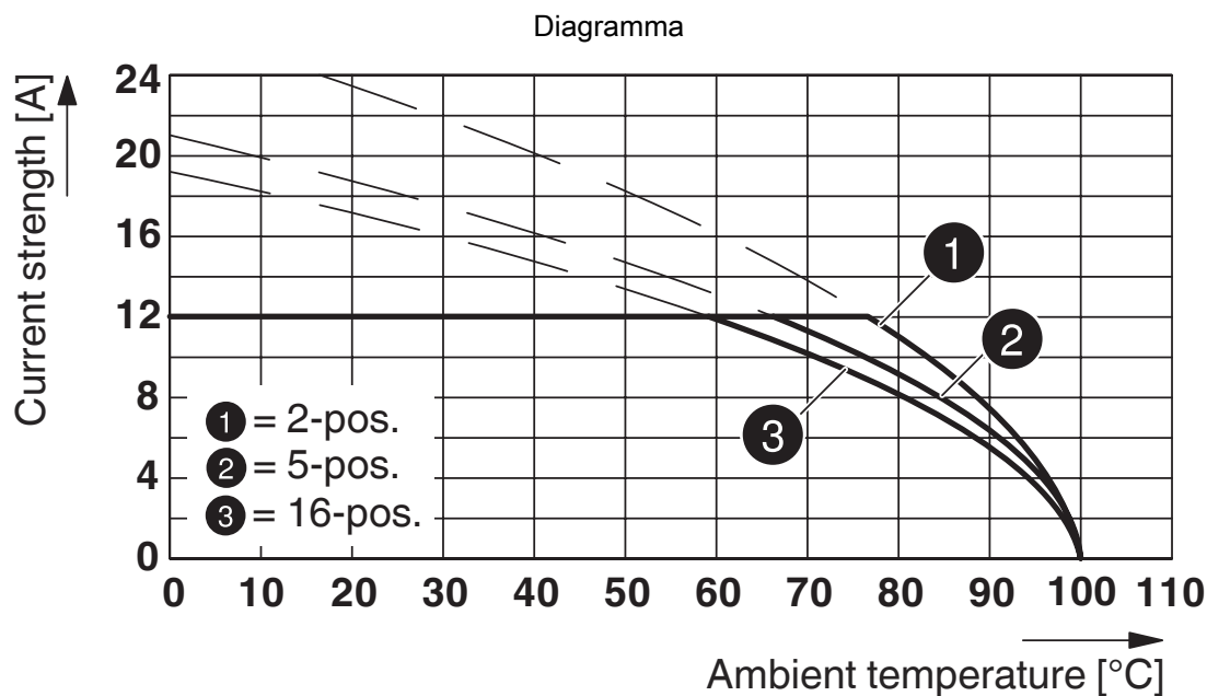
Tipo: FKIC 2,5/...-ST-5,08 con ICV 2,5/...-G-5,08
