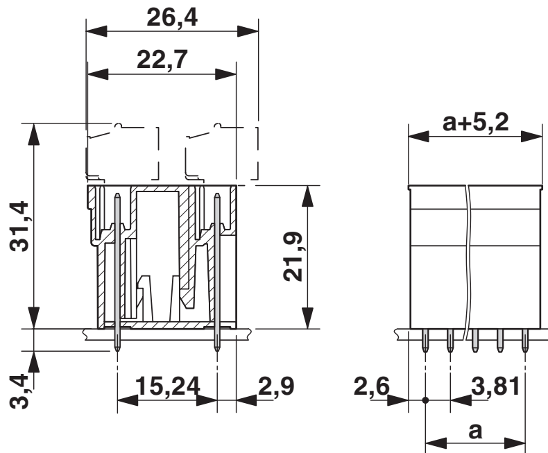
Disegno quotato
