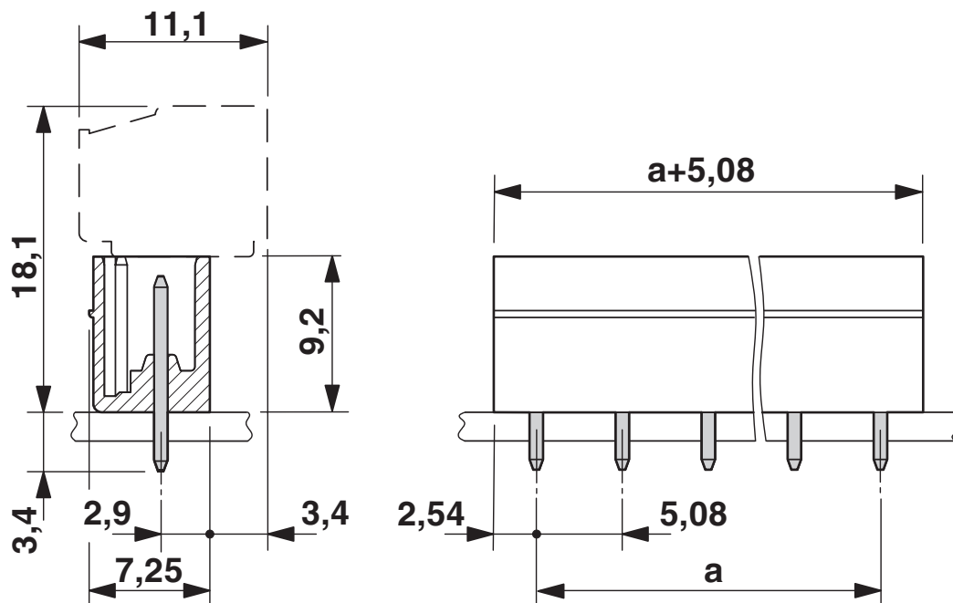
Disegno quotato
