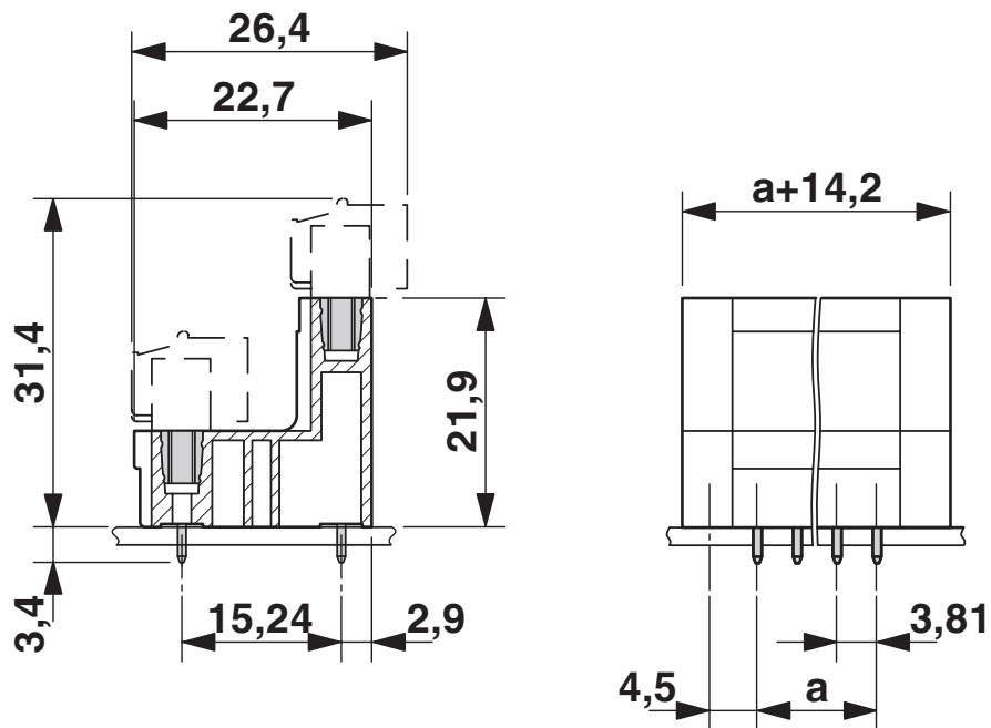
Disegno quotato
