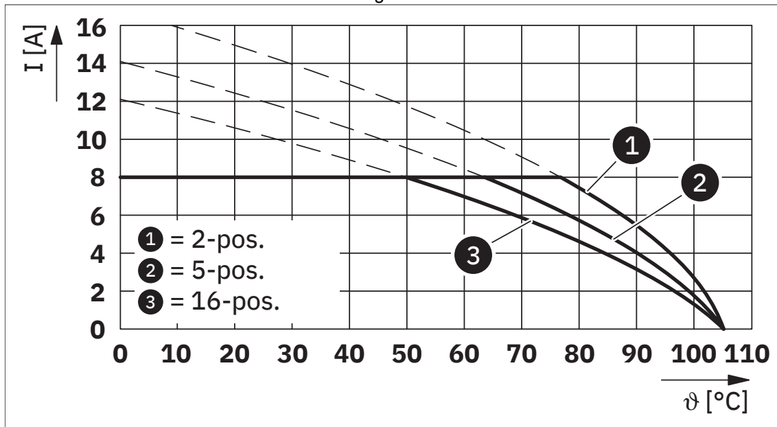
Tipo: FMCOR 1,5/...-ST-3,5 con MC 1,5/...-G-3,5 P... THR
