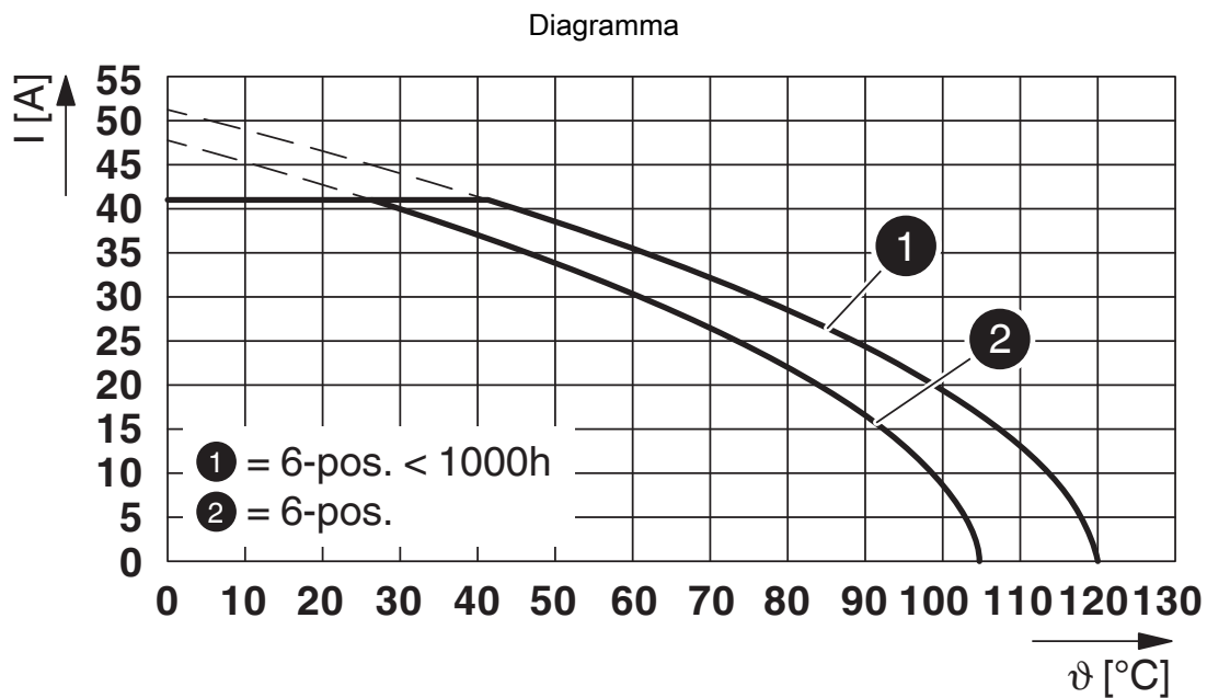
Tipo: LPC 6/...-STL...-7,62 con PC 6/...-GL...-7,62 P...THR
