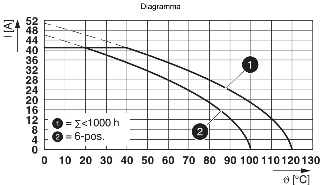
Tipo: LPC 6/...-STL...-7,62 con PCV 6/...-GL...-7,62
