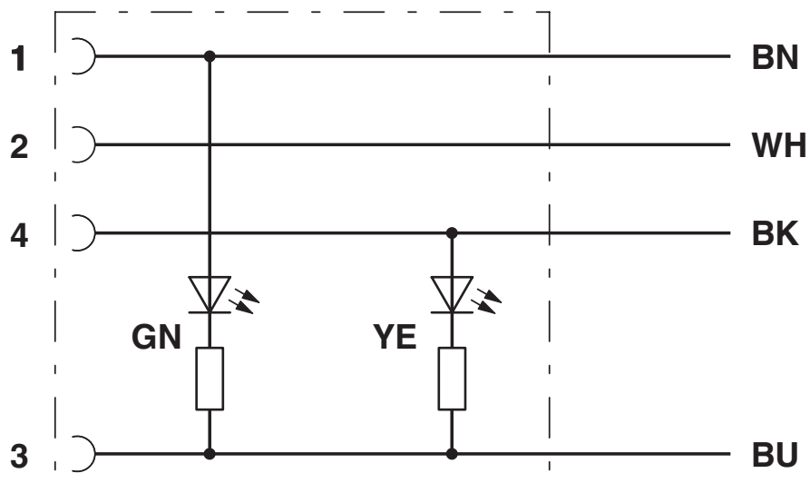
Equipaggiamento dei contatti dei connettori femmina M8/M12 con LED
