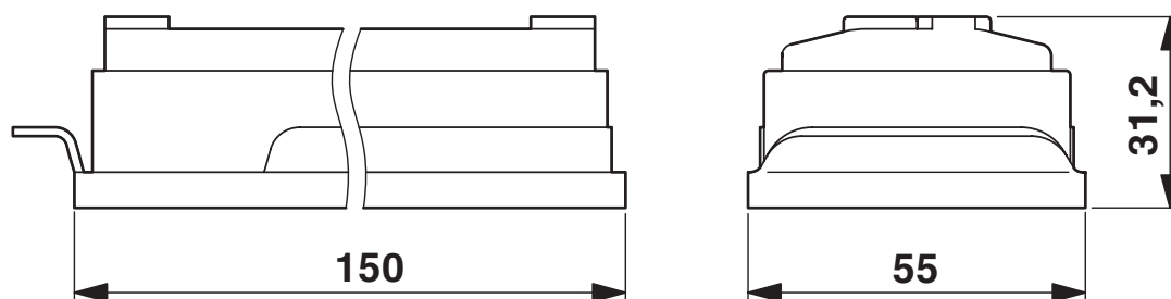
Disegno quotato
