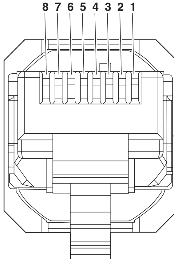
Disegno schema
