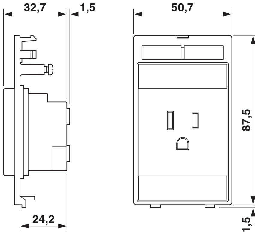
Disegno quotato
