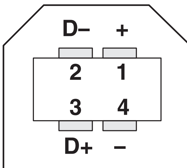
Disegno schema
