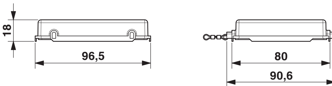
Disegno quotato
