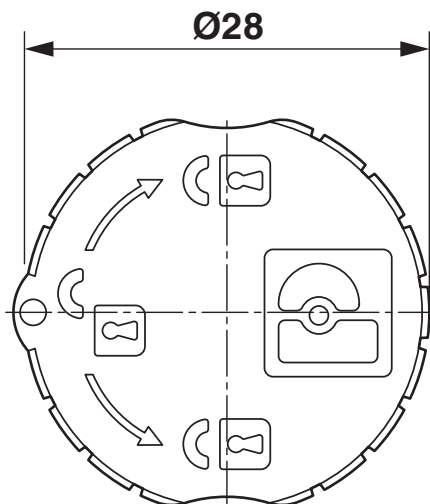
Disegno quotato
