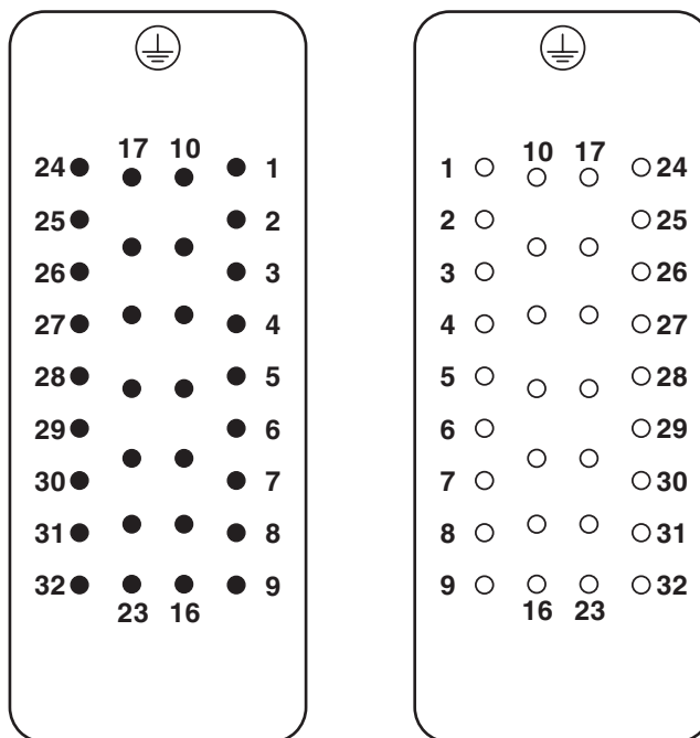
Disegno schema
