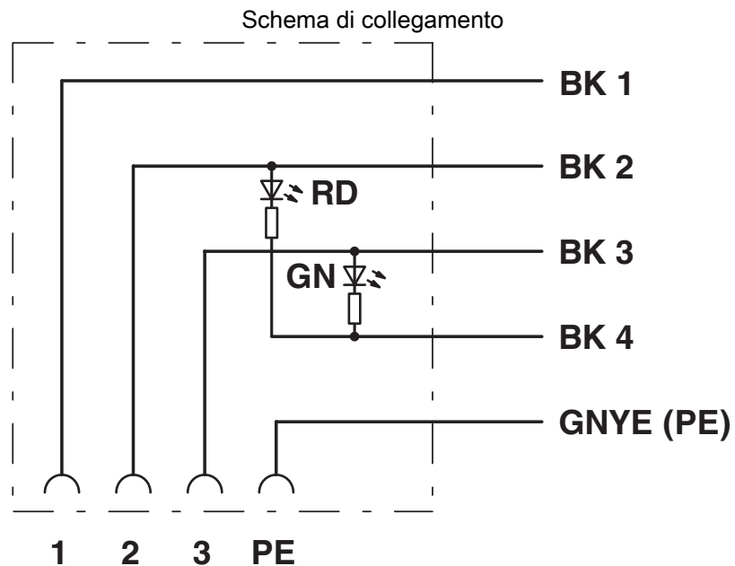
Equipaggiamento dei contatti del connettore per valvole
