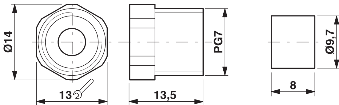
Disegno quotato
