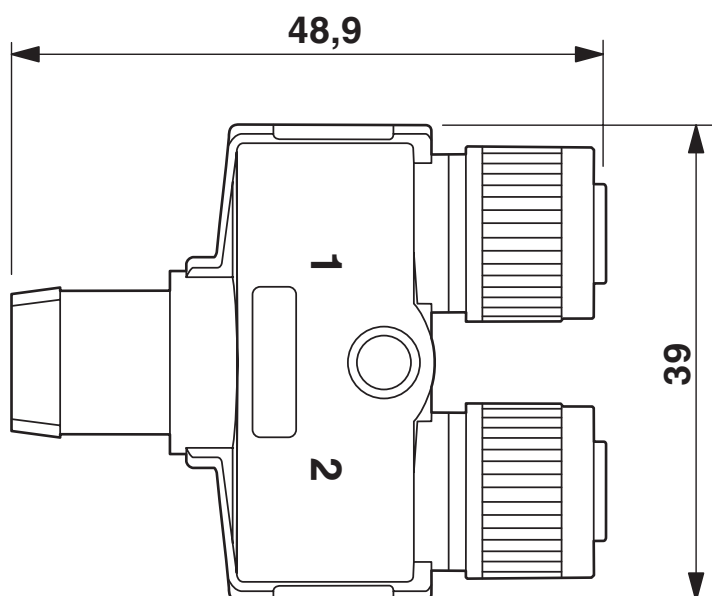
Disegno quotato
