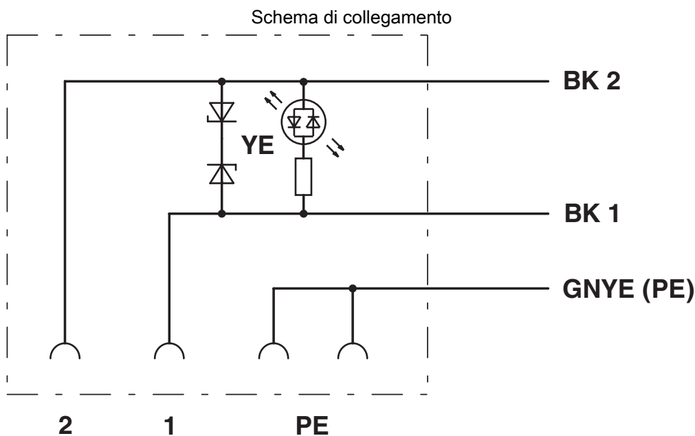
Equipaggiamento dei contatti del connettore per valvole
