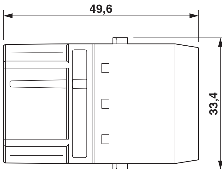
Disegno quotato
