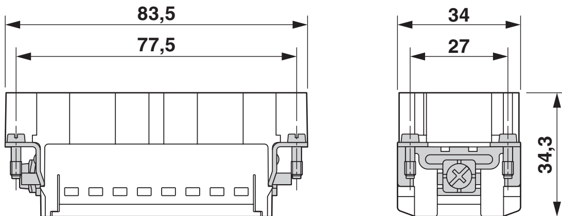
Disegno quotato
