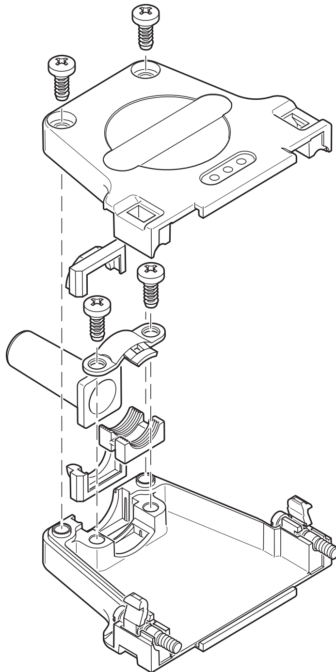
Disegno schema
