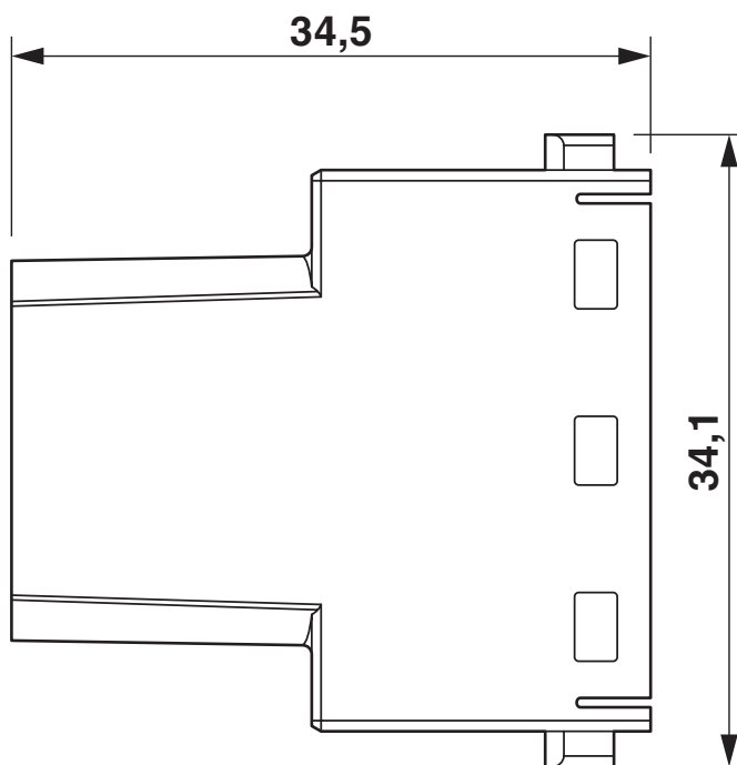
Disegno quotato
